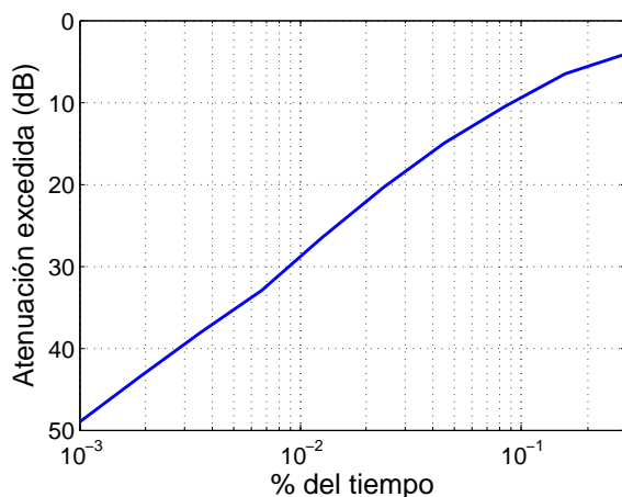
Figura 5.1 Atenuación por lluvia excedida en el p % del tiempo para 13 GHz y 15 km de distancia.
